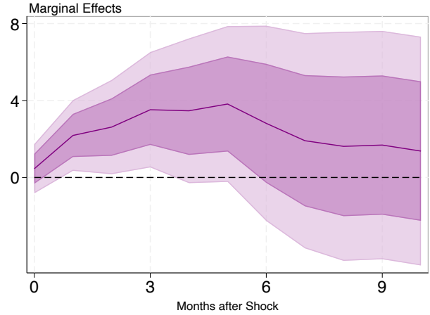
(D) Below 50 th EBP_{ikt-1} Percentile
