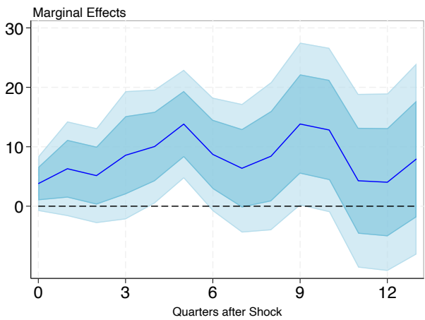
(D) Below 33 rd EBP_{it-1} Percentile
